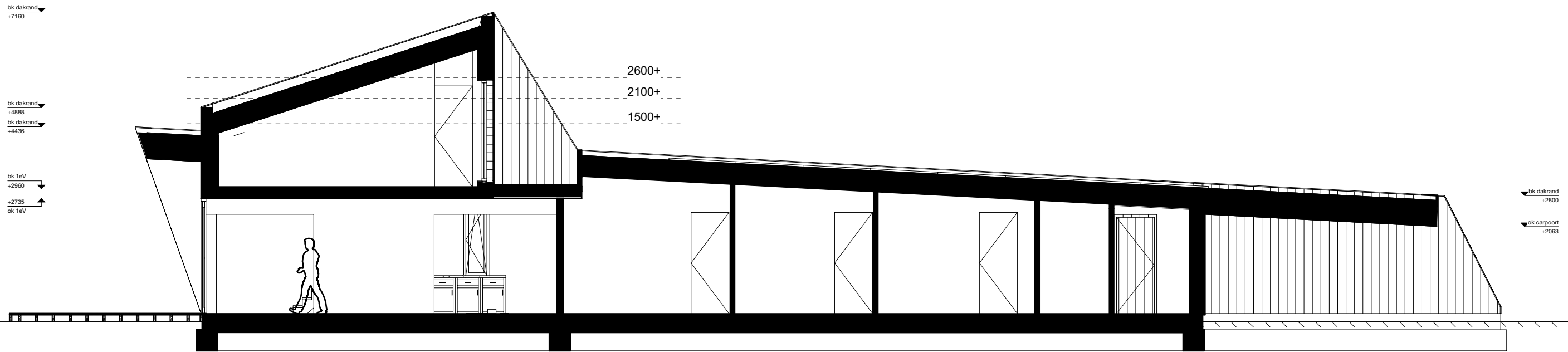
Doorsnede A-A
