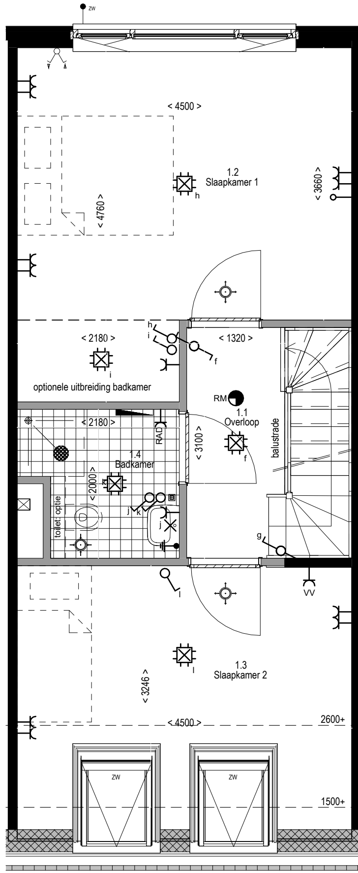
Eerste verdieping - BNR 03
