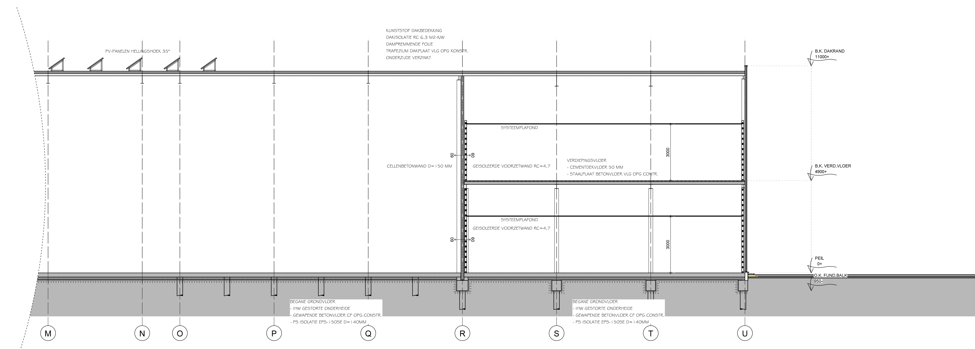
Doorsnede C-C
