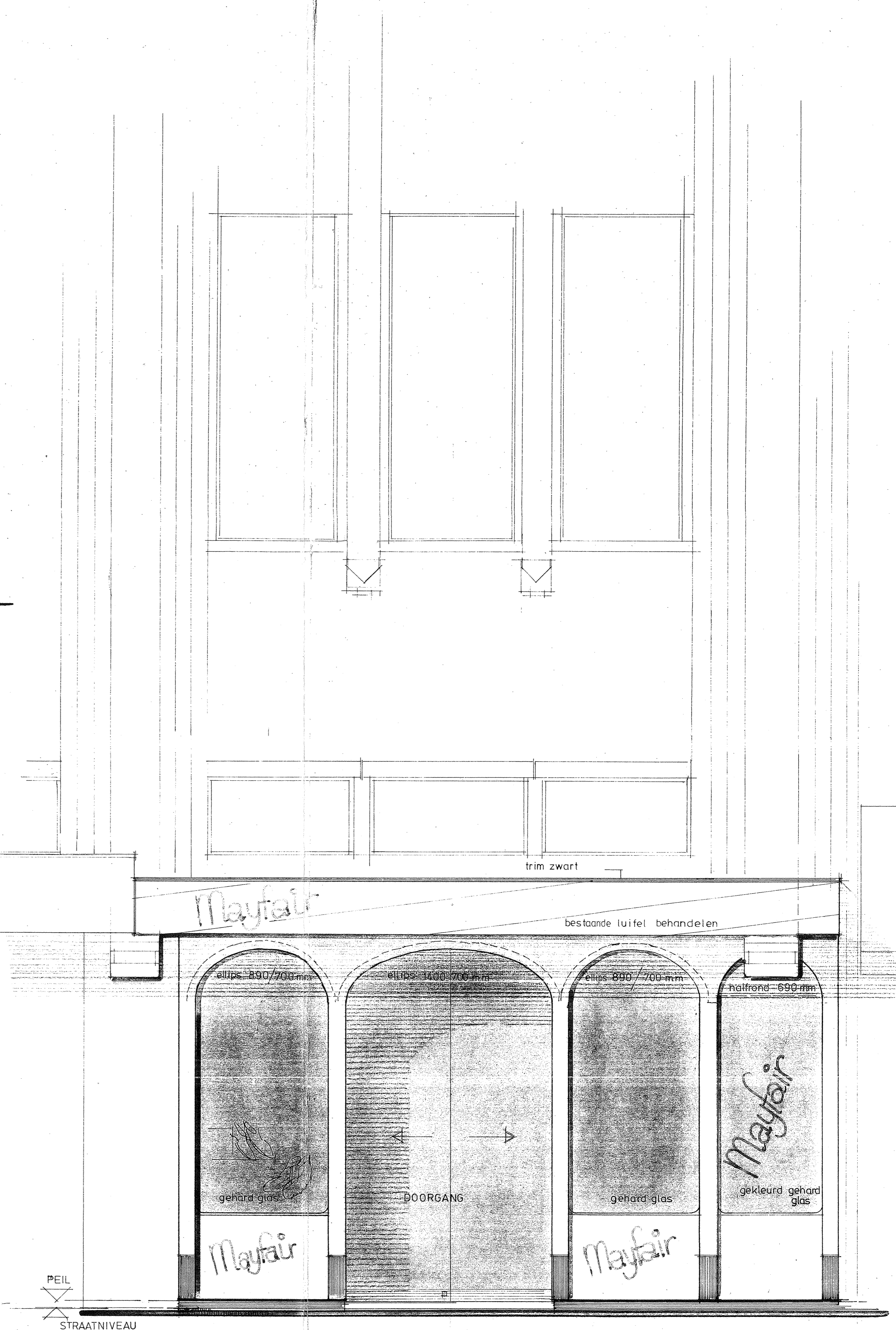
VOORGEVEL
