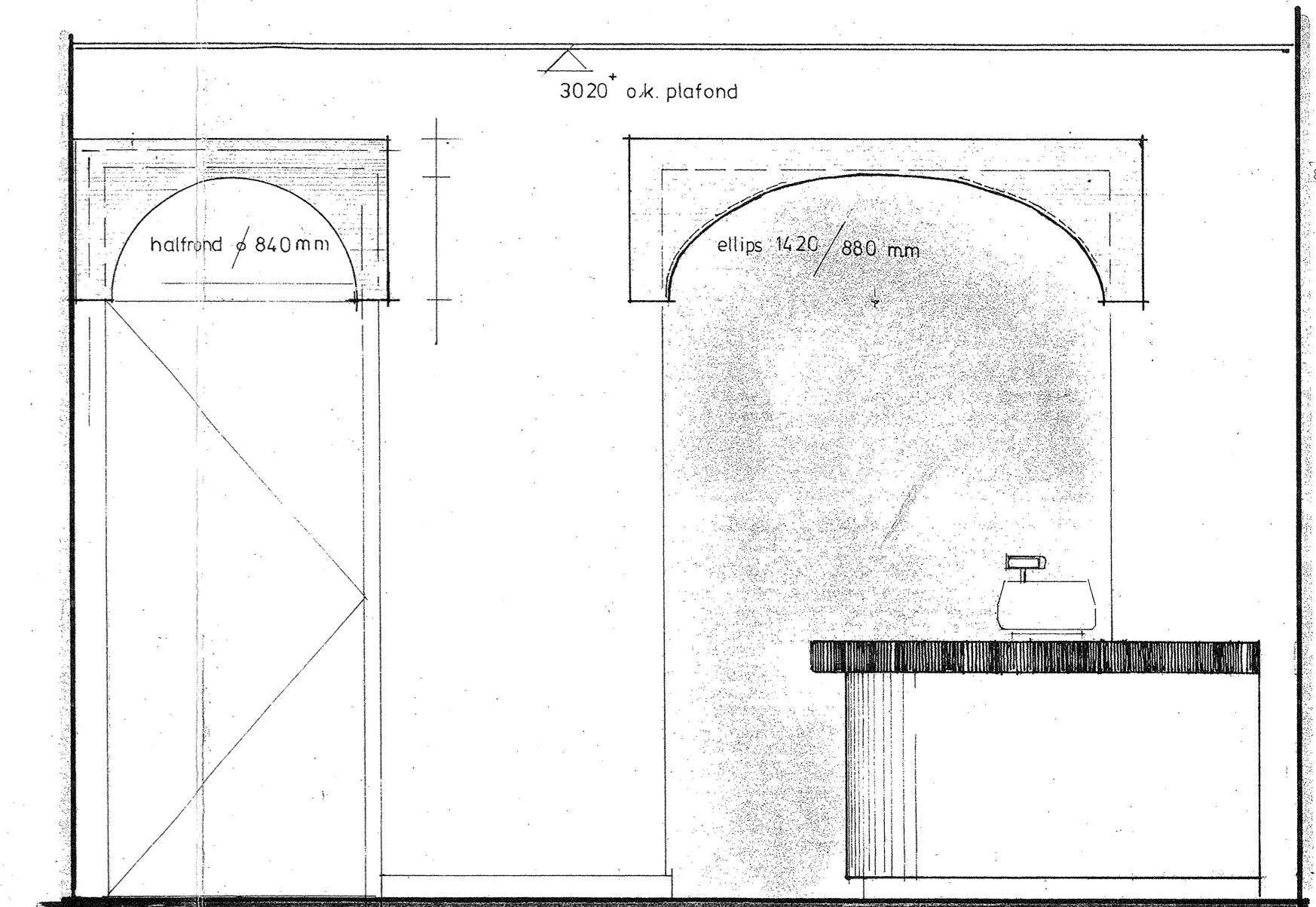
WANDAANZICHT C
