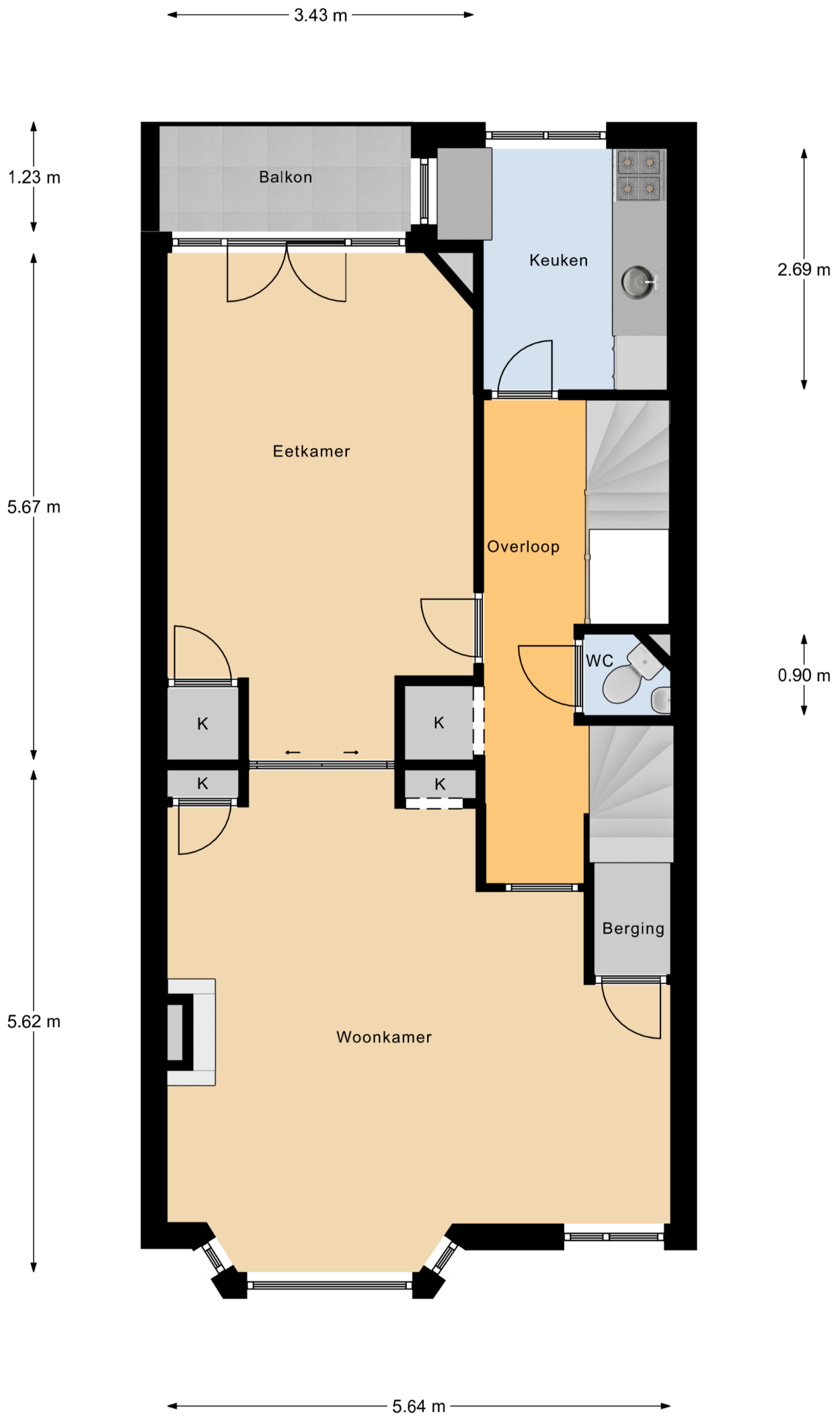
2e Verdieping
