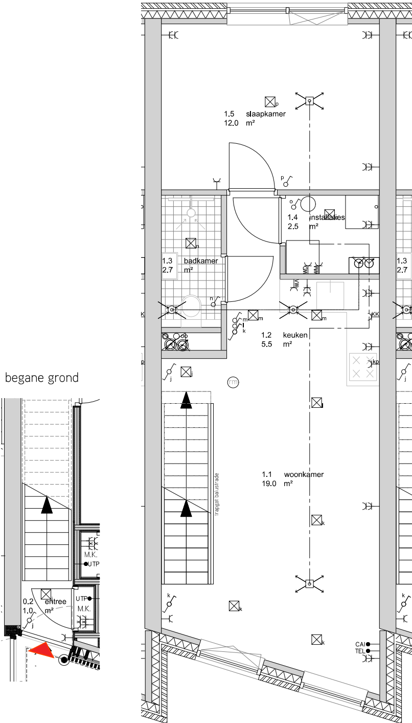
1e verdieping
