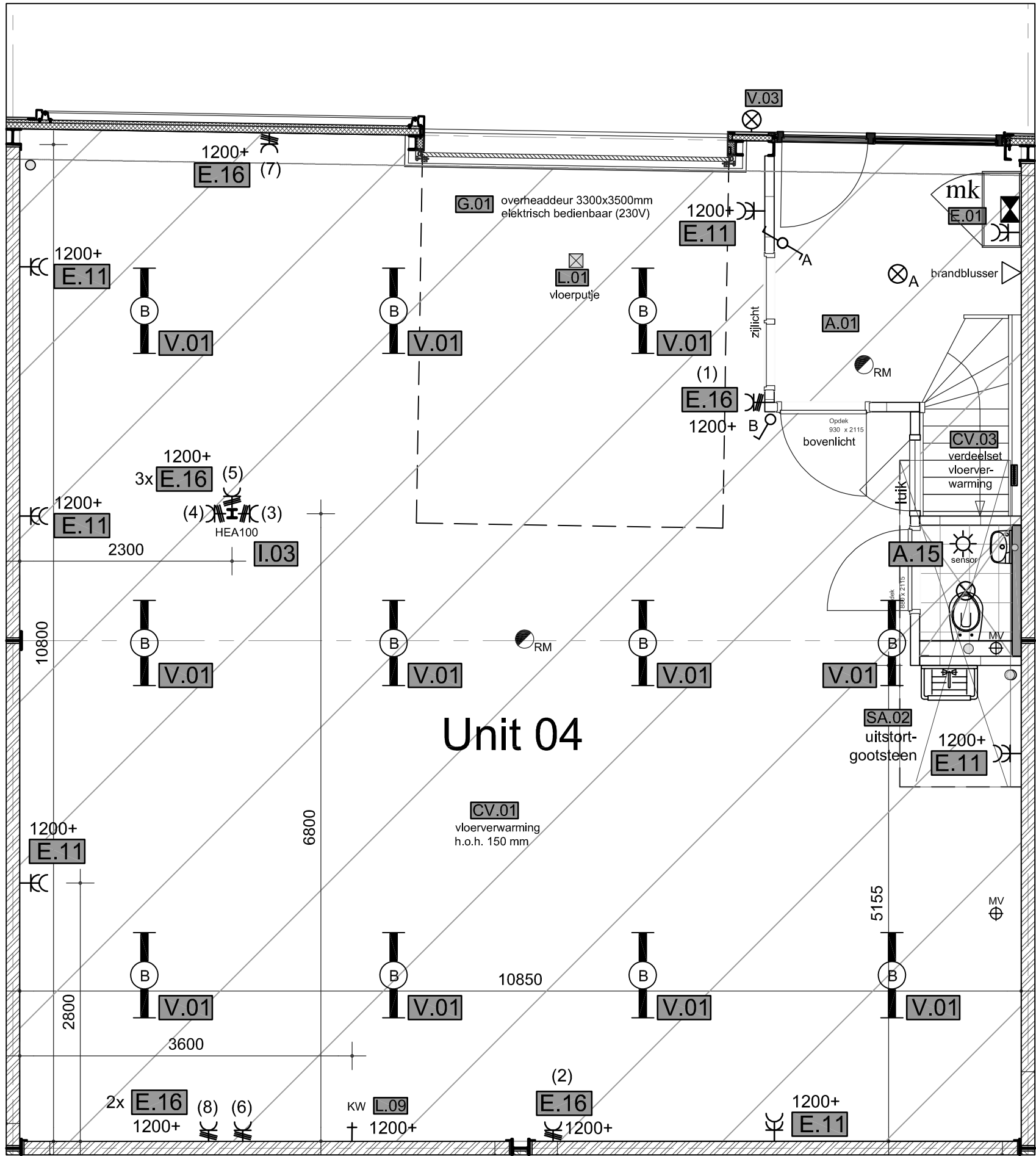
Begane grond
