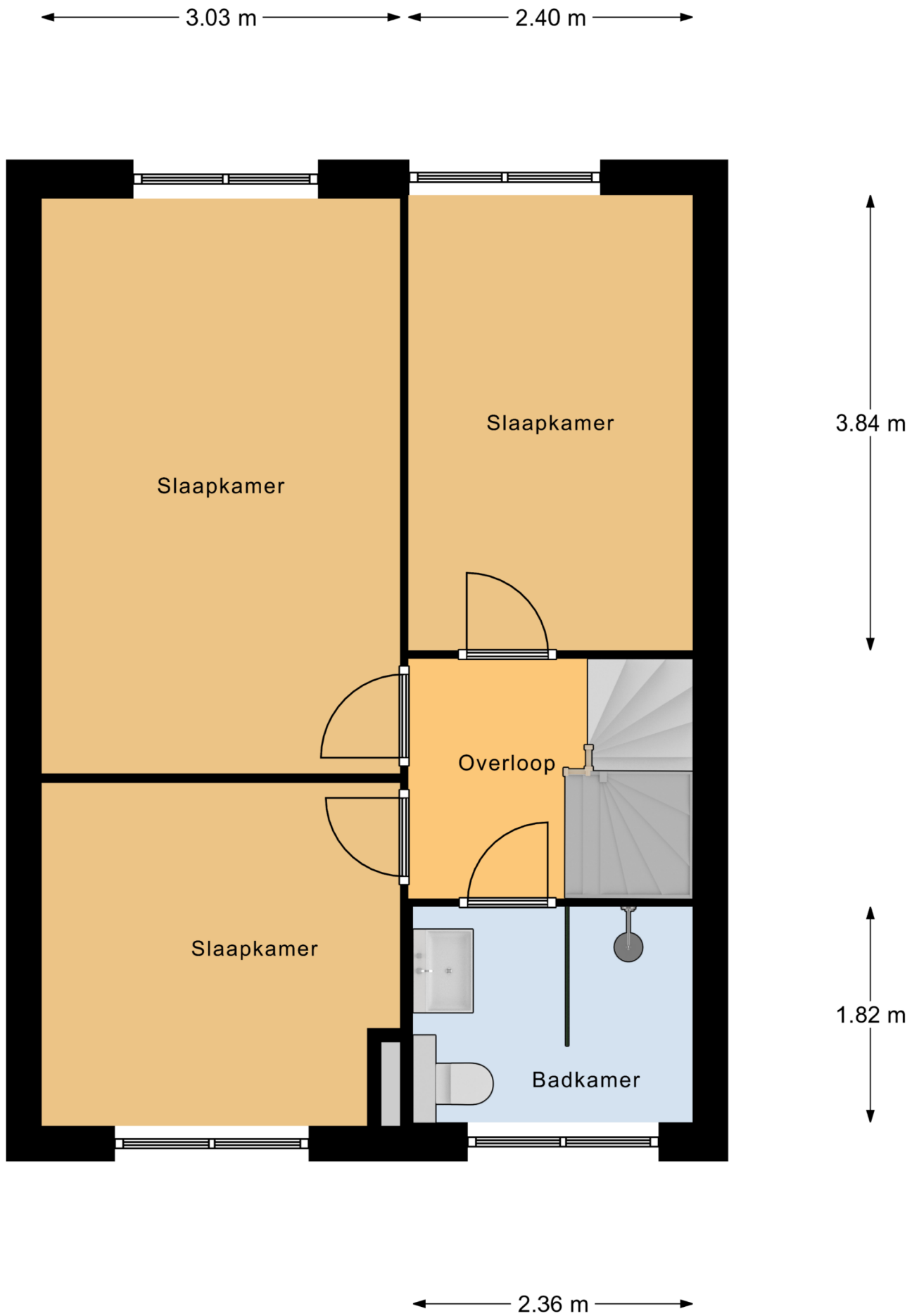
1e Verdieping
