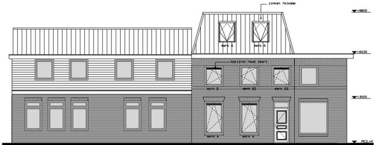
VOORGEVEL
