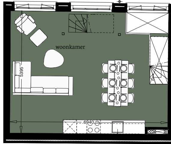
verdieping een
