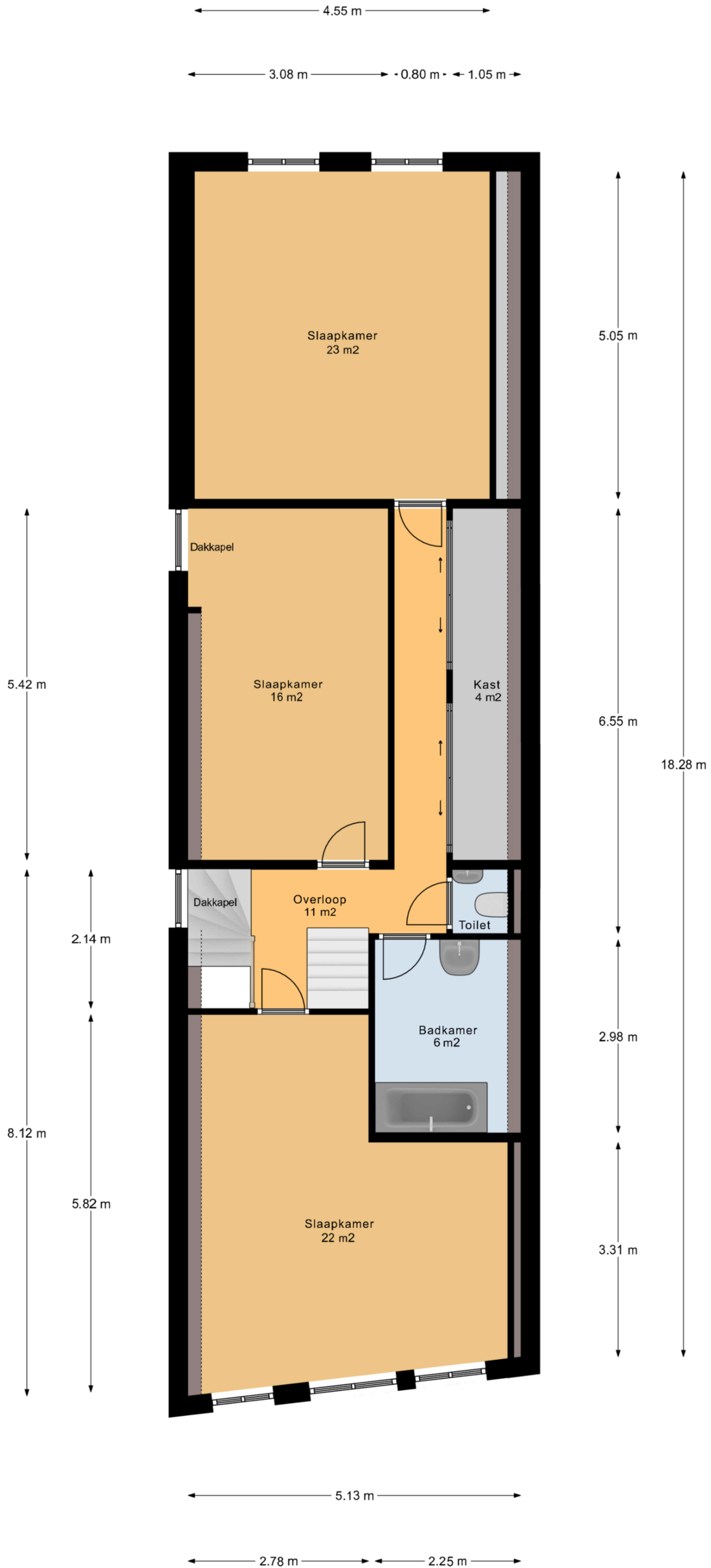
2e Verdieping
