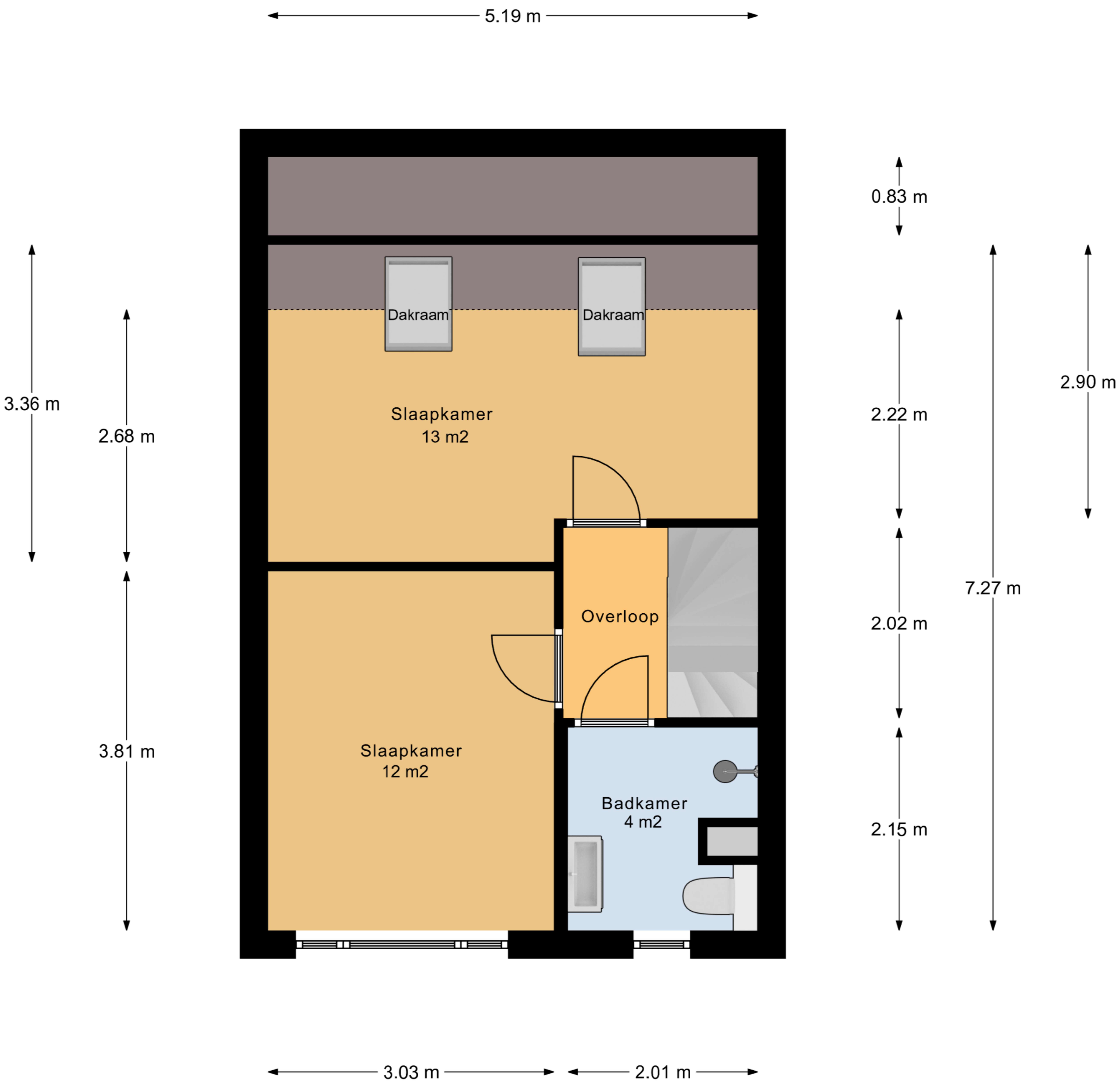
1e Verdieping
